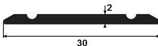
A6227 0,147 kg/m
