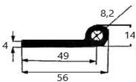
A4714 (zawiasowy) 0,76 kg/m
