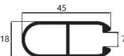
A6062 0,49 kg/m
