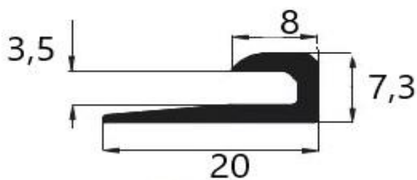
S 73004 0,14 kg/m
