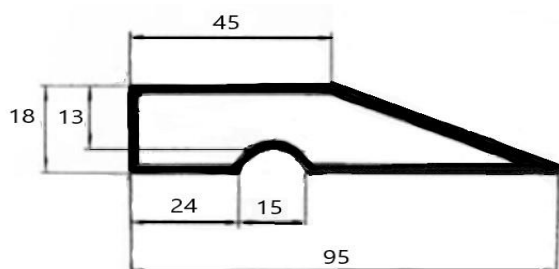
A6322 (tata murarska) 0,85 kg/m
