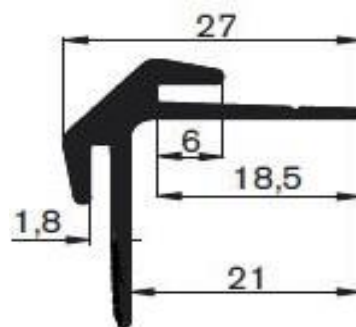
S 73002 0,3 kg/m
