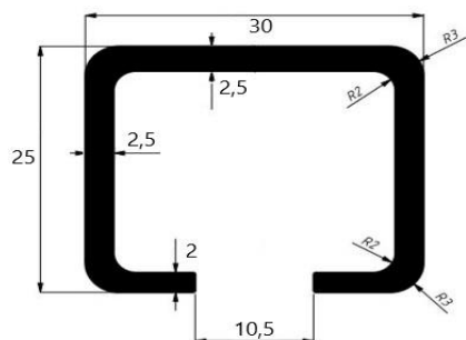
A8526 0,57 kg/m
