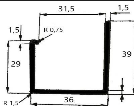
A4672 0,41 kg/m
