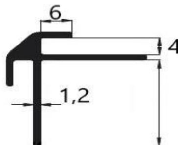
S 73005 0,24 kg/m
