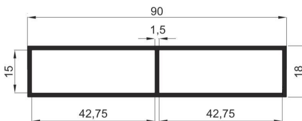
A 6085 (tata murarska) 0,92 kg/m
