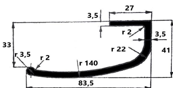
A2874 (antaba) 1,43 kg/m
