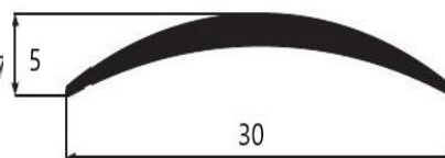
A6280 0,127 kg/m
