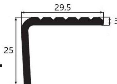
A2581 0,45 kg/m
