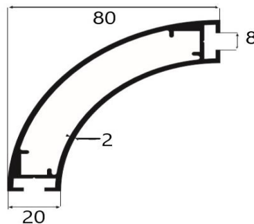
A 6134 0,55 kg/m
