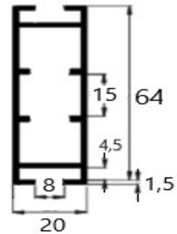
A 6038 0,79 kg/m
