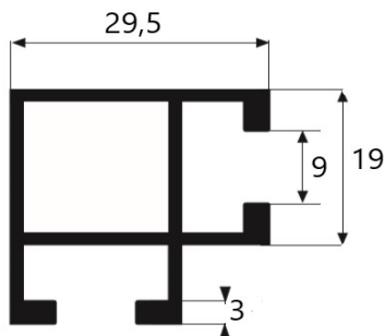
A 4857 0,58 kg/m
