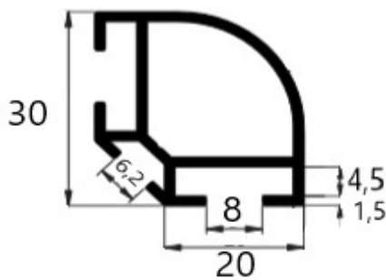
A 6036 0,55 kg/m
