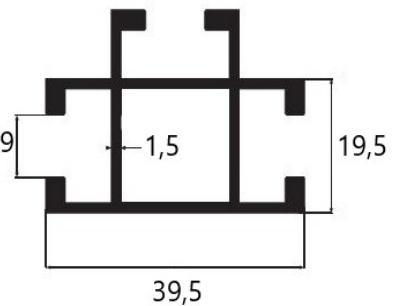
A 4856 0,72 kg/m
