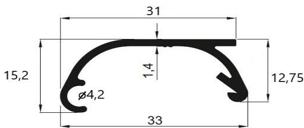
A 6036 0,55 kg/m
