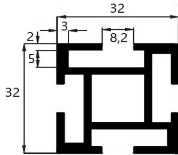
A 4215 0,98 kg/m
