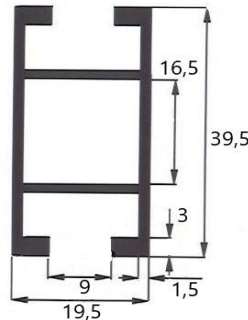
A 4858 0,58 kg/m
