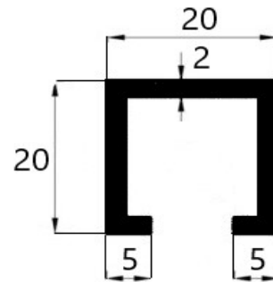
A 4543 0,34 kg/m
