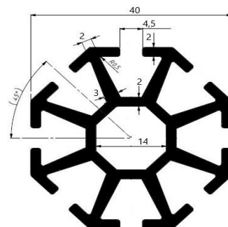
A 6248 1,3 kg/m
