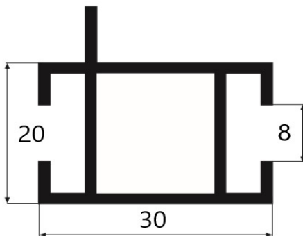
A 6074 0,23 kg/m
