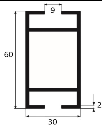
A 5642 1,11 kg/m
