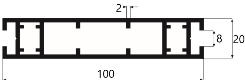
A 6133 1,64 kg/m
