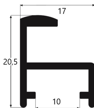
A 4858 0,58 kg/m
