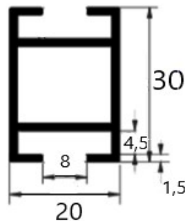
A 6037 0,45 kg/m
