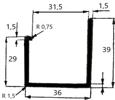
A 4672 0,41 kg/m
