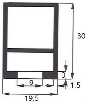
A 3611 0,44 kg/m
