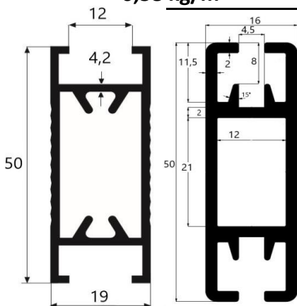
A 5087 0,68 kg/m
