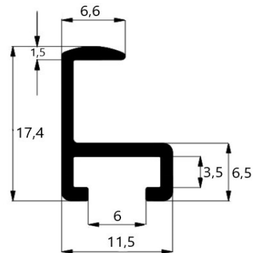
A 6212 0,14 kg/m
