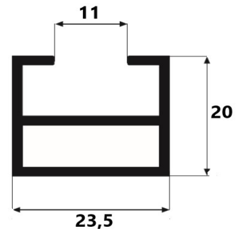
A 4933 0,37 kg/m
