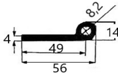
A 4714 0,76 kg/m
