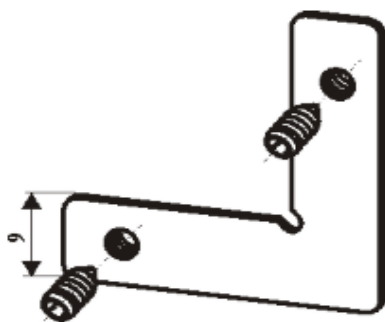
kątownik do A6212 10-04-057
