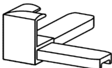
głowica do A 6212 10-04-689
