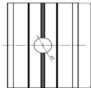
90338 (1) 0,519 kg/ mb
