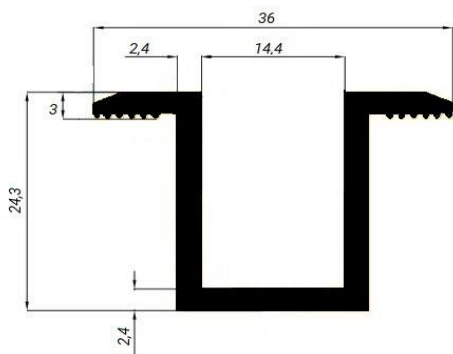
90338 0,519 kg/ mb
