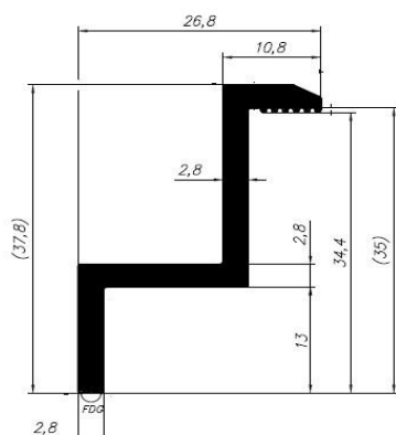
90433 0,446 kg/mb
