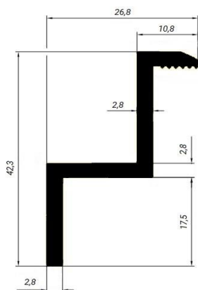
90339 0,50 kg/mb
