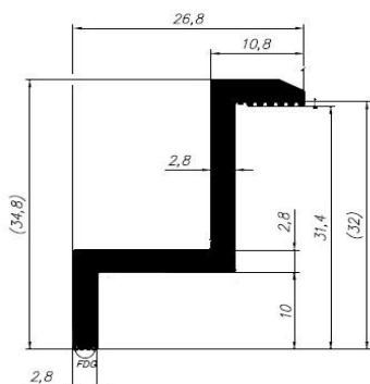
90432 0,444 kg/mb
