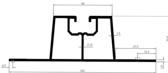
90444 0,983 kg/mb
