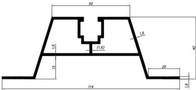
6148 1,201 kg/mb
