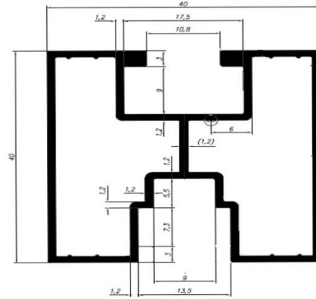
90435 0,806 kg/mb
