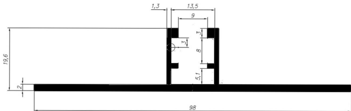
90454 0,707 kg/mb
