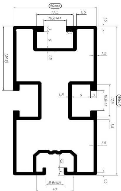
90443 1,55 kg/mb
