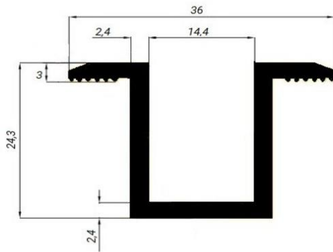
90338 0,519 kg/ mb
