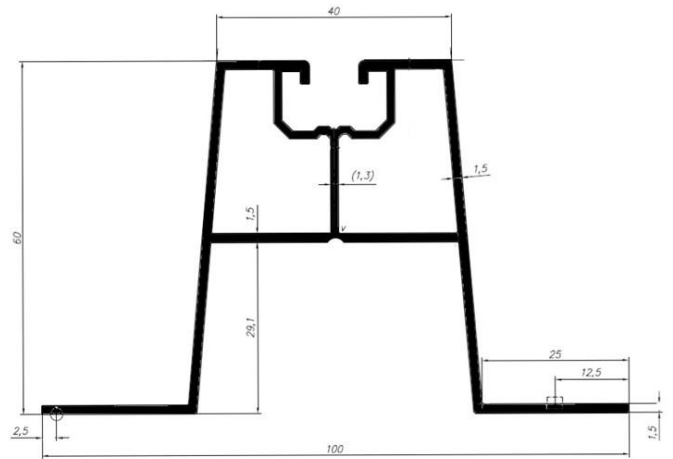
90445 1,199 kg/mb
