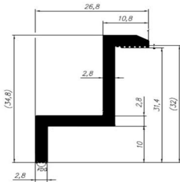
90432 0,444 kg/mb
