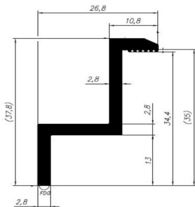
90433 0,446 kg/mb
