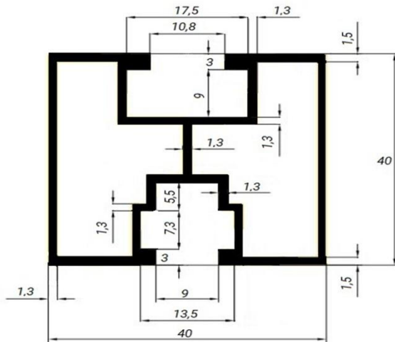
90337 0,886 kg/mb
