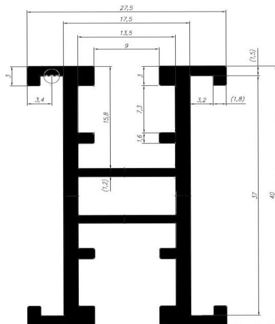
90453 0,741 kg/mb
