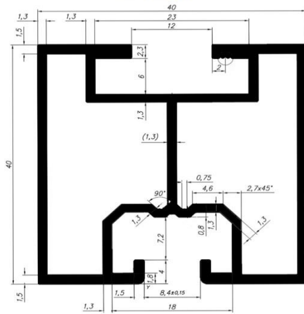
90440 0,888 kg/mb
