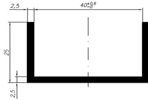
90431 0,607 kg/mb
